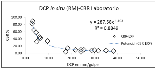
Fig. 6 Grafica del DCP in situ RM-CBR Laboratorio
