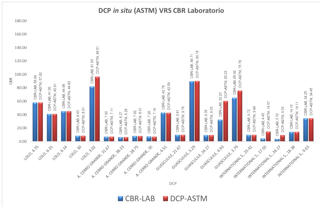
Fig. 8 Grafica CBR ASTM Vs CBR Experimenta
